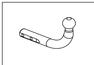
KULA TYP S Kula stała, przykręcana za pomocą dwóch śrub M12
